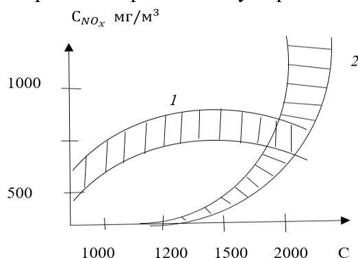
1-расм. Ҳароратнинг ошиб бориши билан азот оксидларининг ҳосил бўлиши. 1-ёқилғи таркибидаги азотнинг, NO_x га айланиши; 2-ҳаво таркибидаги азотнинг, NO_x га айланиши.
