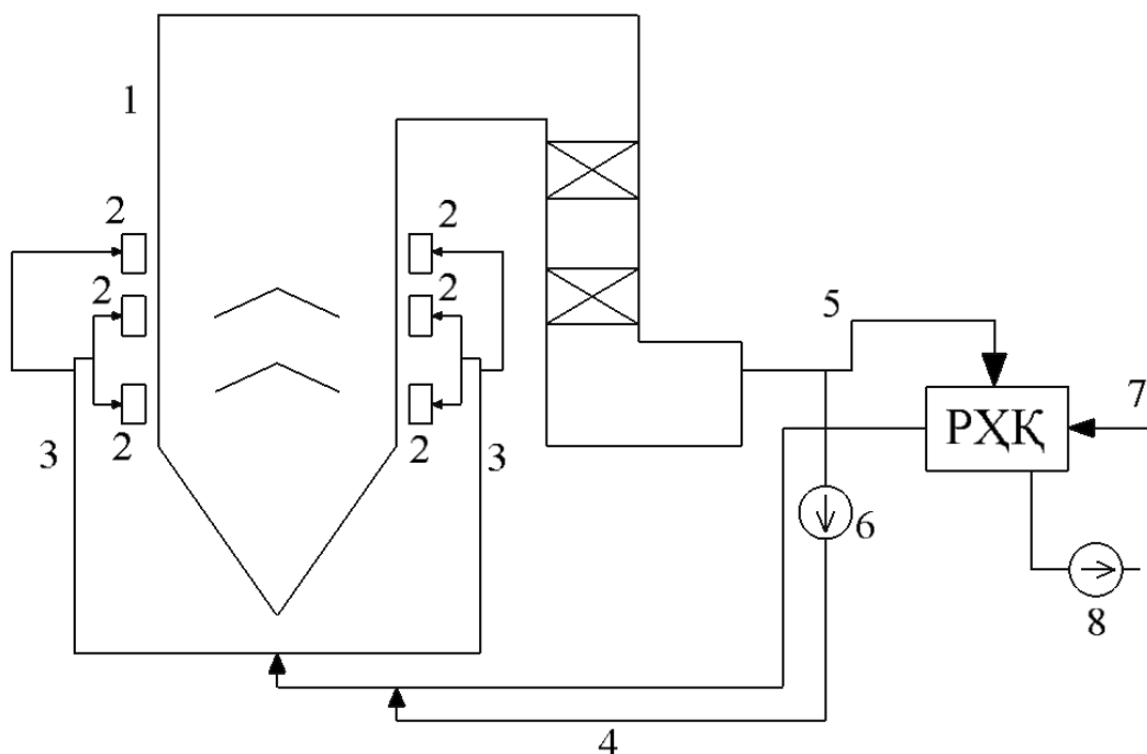
5-расм. Ёқилгани уч босқичга ёқиш ва тутун газини рециркуляция қилиш схемаси.
