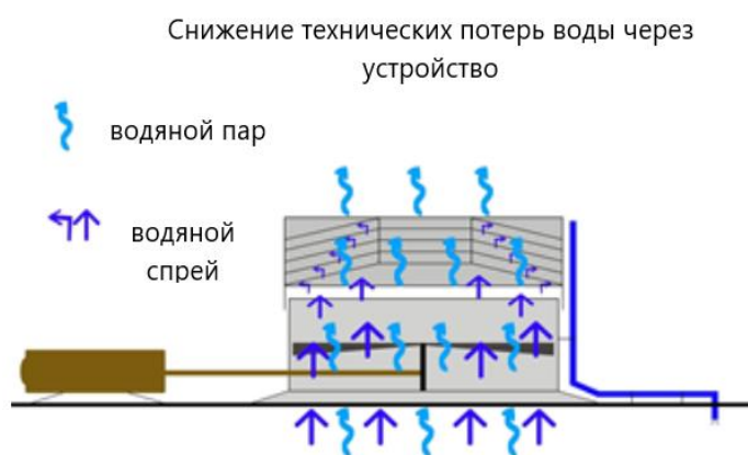
5 рисунок. Технологическая схема улавливания воды
