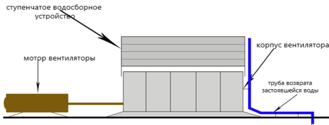
2 рисунок. Технологическая схема улавливания воды
