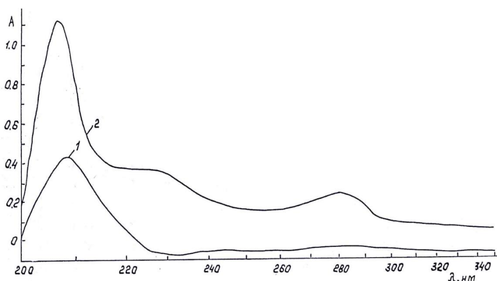
Рис.3.УФ-спектры:1-карбамид; 2- C_7H_6N_2O
