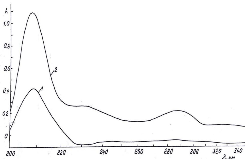
Рис.4.УФ-спектры:1-карбамид; 2- C_7H_5N_2OCl
