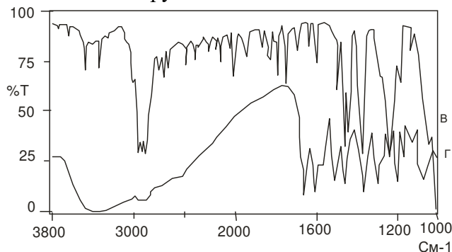
Рисунок 2. В-ИК-спектр уротропина; Г-спектр ПК рутин:уротропин (1:3, 60g).
