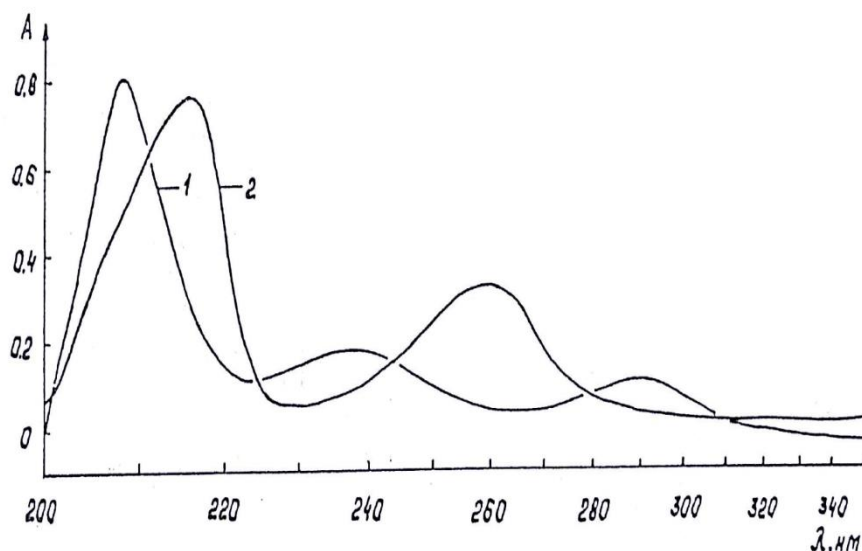
Рис.1.УФ-спектры:1-Карбамид, 2- \text{C}_7\text{H}_9\text{NO}
