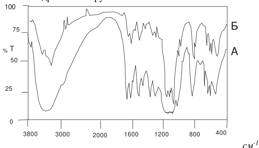
Рисунок 1. А - ИК-спектр ПК рутин: \text{FeSO}_4 (1:1, 60g); Б - спектр вычитания спектров ПК рутин: \text{FeSO}_4 (1:1, 60g) и рутина.
